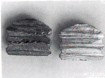
Dwarsdoorsnede kogels. Links lood, rechts bismut.
