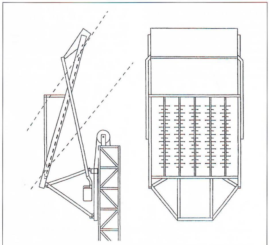
Een voorbeeld van de kogelvanger met een doorzichtige achterwand, zoals deze door de Limburgse schutterijen gebruikt kan worden (Jansen Products). Afbeelding 16 uit de Circulaire "Traditioneel schieten" 1999.
